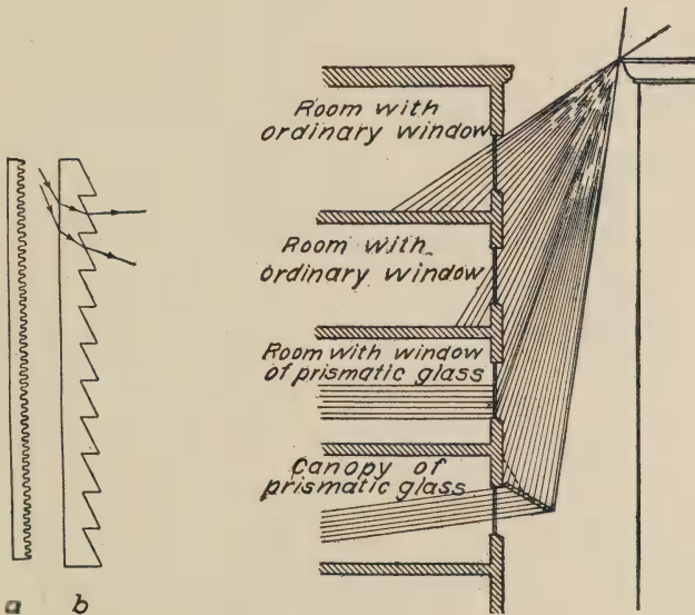
FIG. 27. PRISM GLASS.
